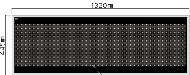
正面 LEDパネル 128×32 (4096個)
